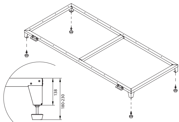
Abb. 6. Montagerahmen des Geräts mit Stellfüßen (muss separat bestellt werden)
