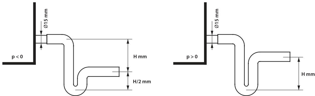
Abb. 13. Installation eines Siphons
