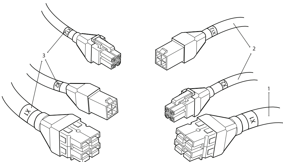
Abb. 24. Kabelverbindungen zwischen Abschnitten
