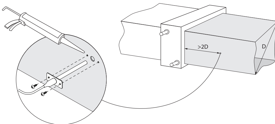
Abb. 21. Installation eines Zulufttemperaturfühlers
