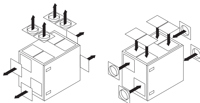
Abb. 2. Verlegung der Kanalanschlüsse der Universalgeräte
