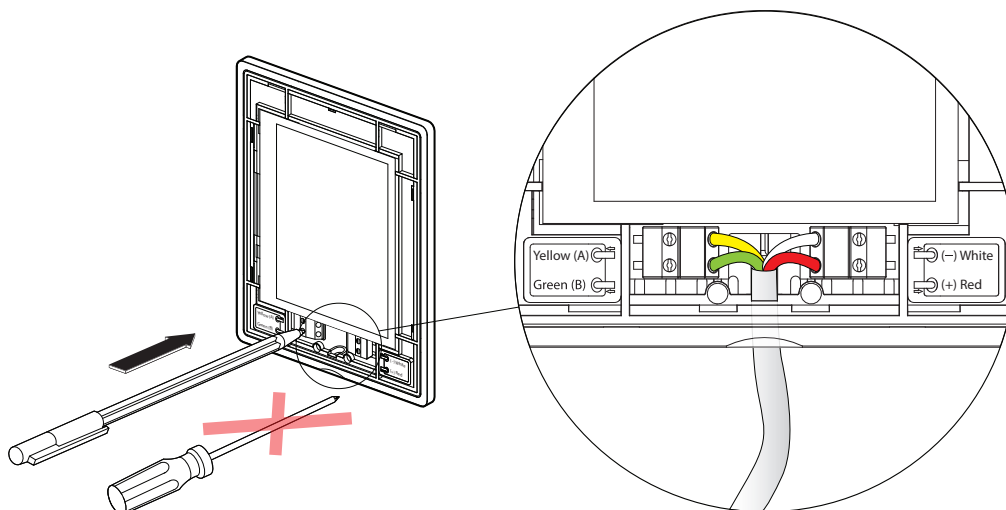
Abb. 23. Anschlussplan für das Bedienpanel
