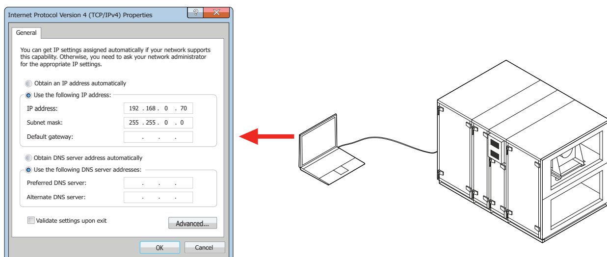
Abb. 26. Computernetzwerkeinstellungen für den direkten Anschluss an das Gerät
