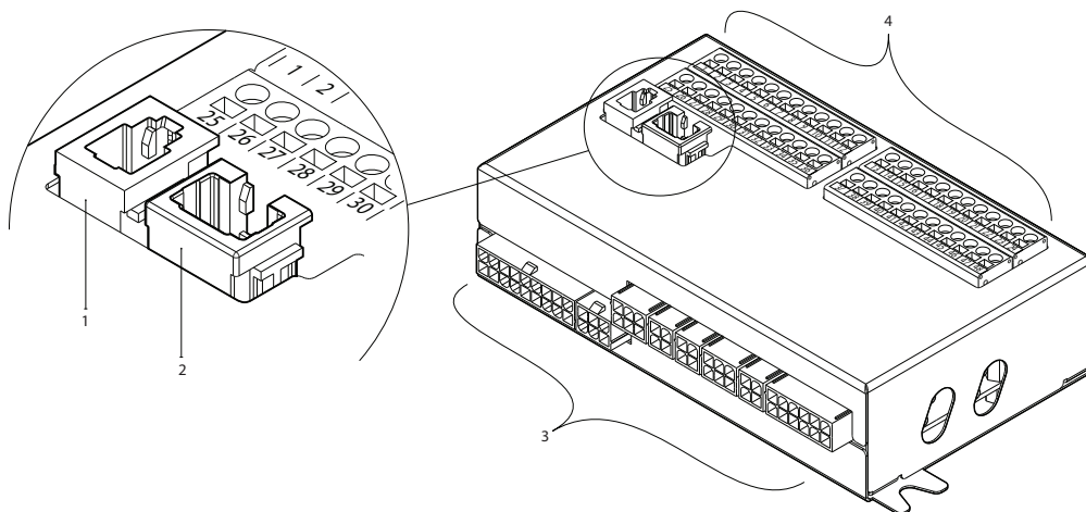
Abb. 17. C5-Steuerung-Hauptboard
