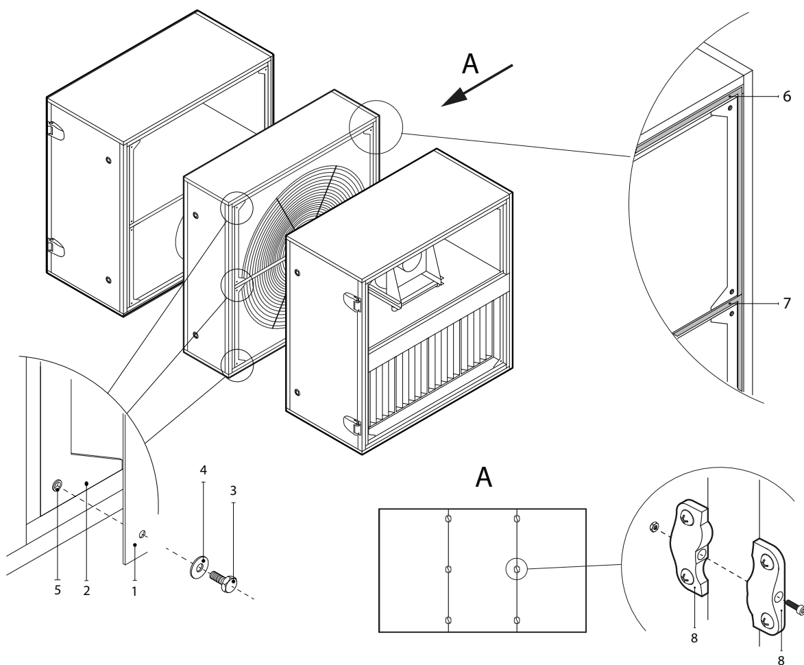
Abb. 10. Verbindung von Abschnitten und deren Abdichtung
