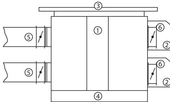
Abb. 16. Zubehör für den Außenbereich 1 - RLT-Gerät, 2 - Hauben, 3 - Dach, 4 - Grundrahmen, 5 - runde Luftklappen (nur für Geräte mit runden Kanalanschlüssen), 6 - rechteckige Luftklappen (nur für Geräte mit rechteckigen Kanalanschlüssen)
