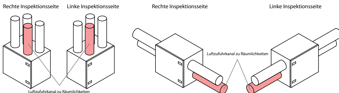
Abb. 3. Klassifikation der Einheiten nach Inspektionsseite
