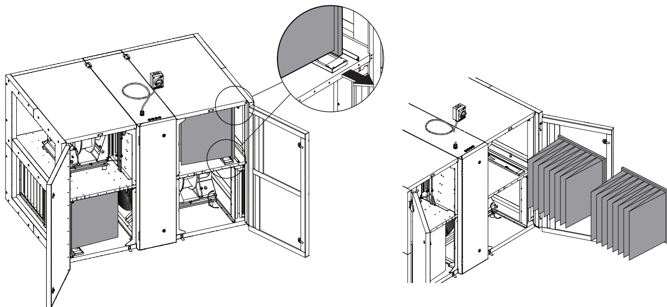
Abb. 29. Ein Beispiel für den Austausch von Beutelfiltern
