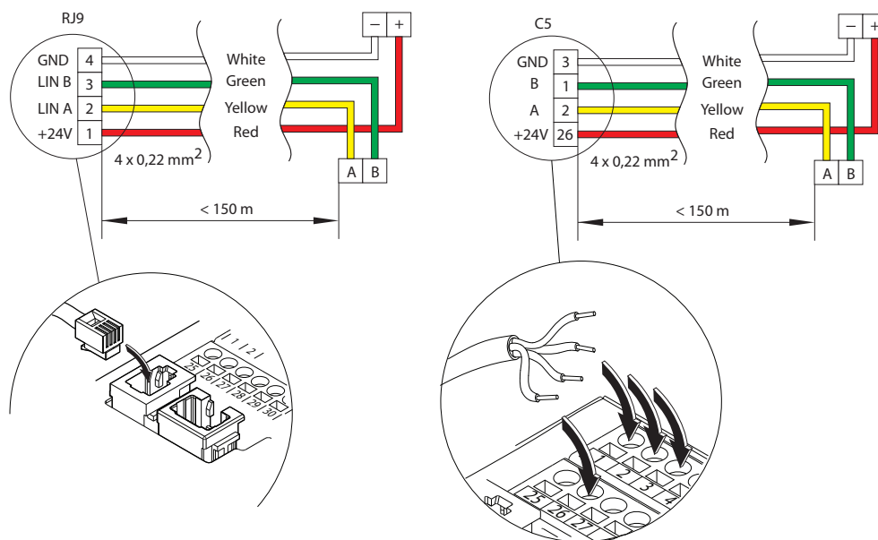
Abb. 22. Anschlussplan für das Bedienpanel
