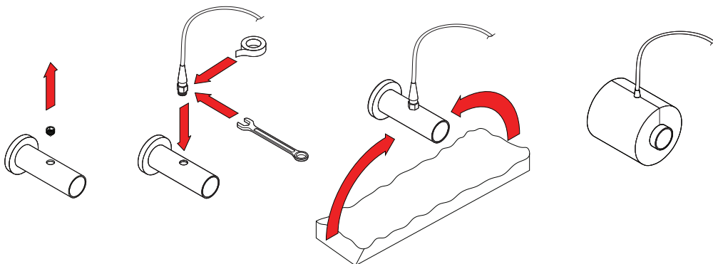
Abb. 12. Installation eines Rücklauf-Wassertemperaturfühlers
