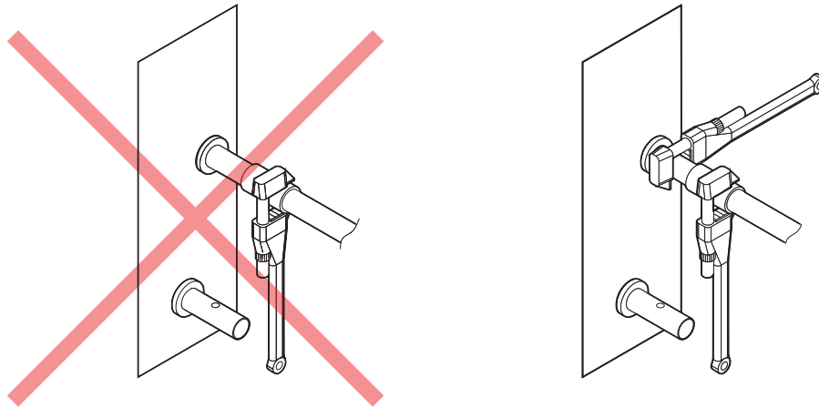
Abb. 11. Anschluss von Muffen
