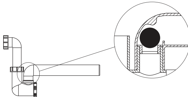
Abb. 14. Beispiel eines Siphons mit Rückschlagventil
