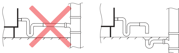
Abb. 15. Anschluss des Kondensatablaufs an die Kanalisation
